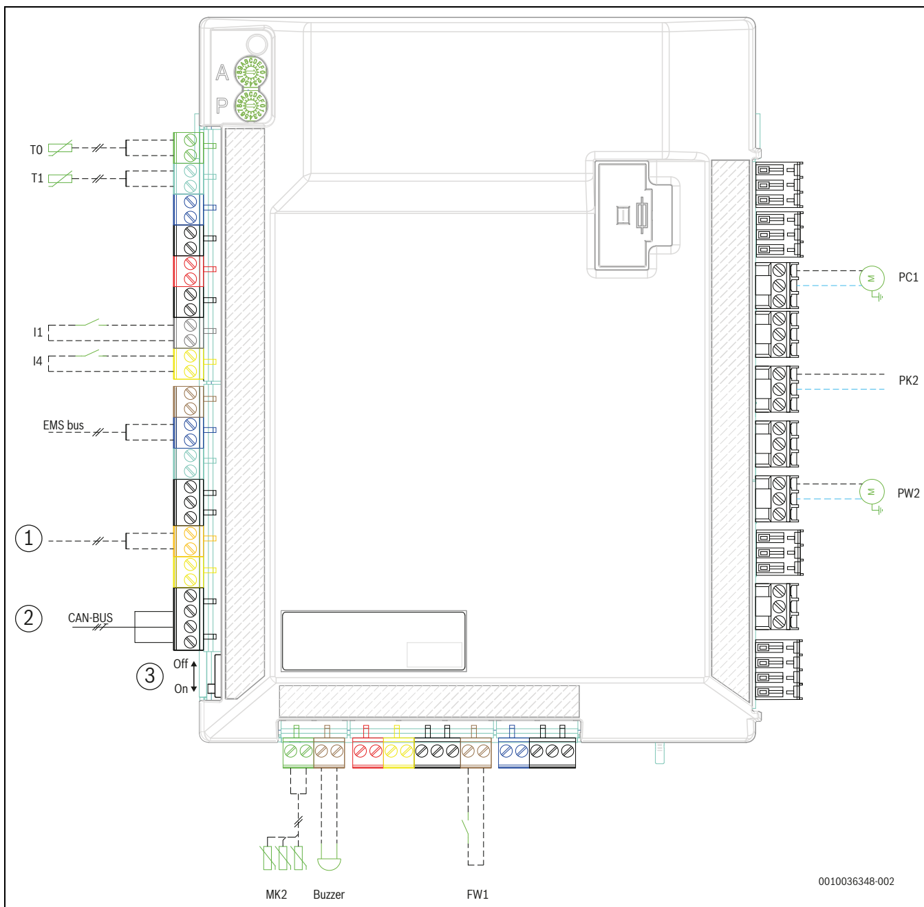
12. ábra A beltéri egység telepítői modulja
