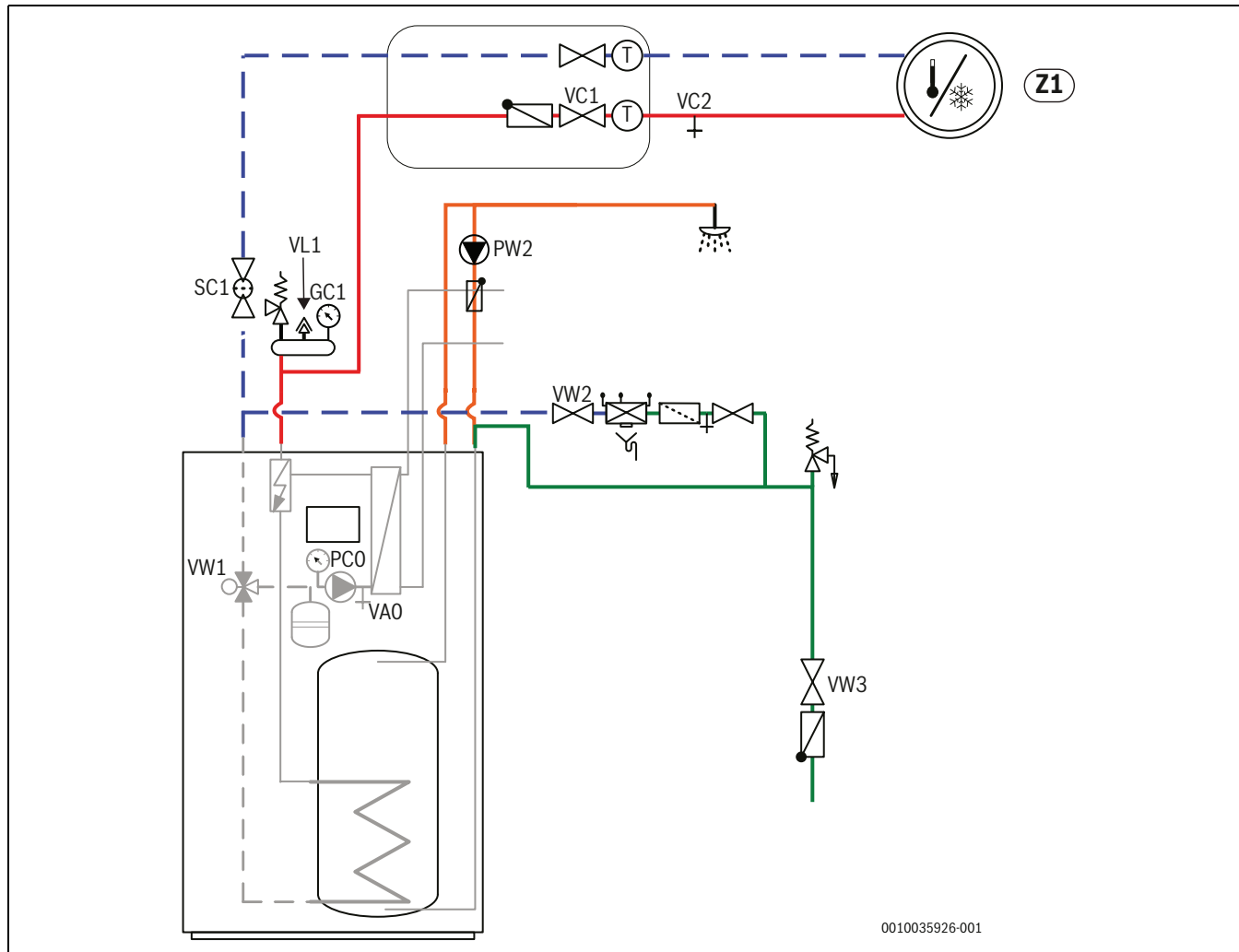
17. ábra A beépített elektromos fűtésrészegítéssel ellátott beltéri egység légtelenítése
