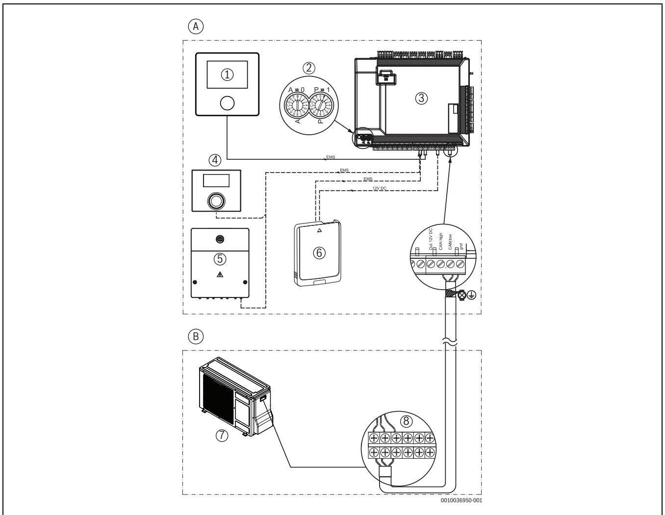
33. ábra CAN-BUS és EMS csatlakozó
