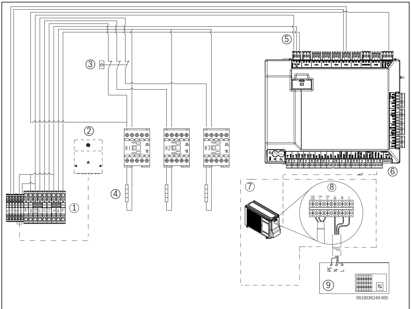
36. ábra 400 V 3N~ beltéri egység, 230 V~ kültéri egységgel
